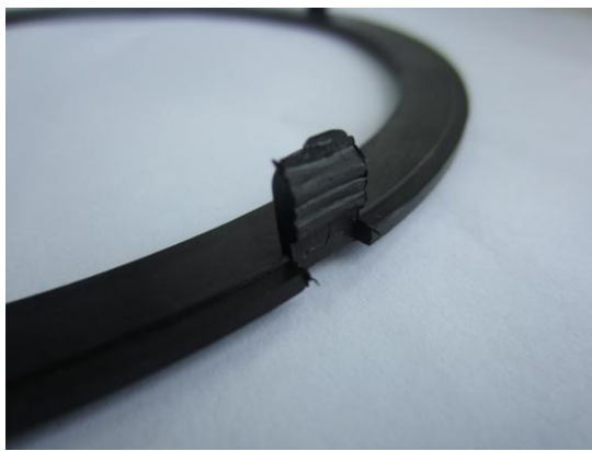
Фото №2.1. Не оригинал: смятые зацепы.
